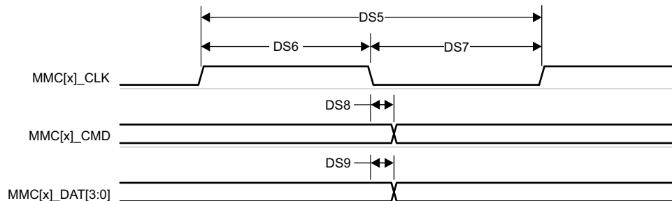
图 7-39. MMC1 - Default Speed - Transmit Mode
