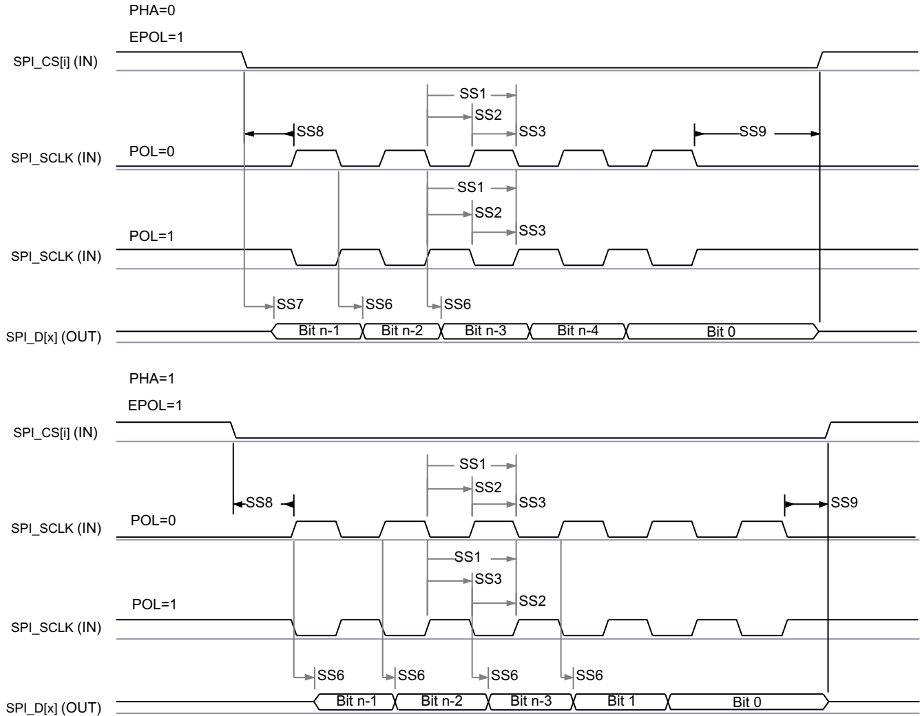
图 7-37. SPI Slave Mode Transmit Timing
