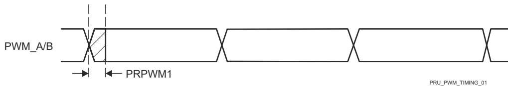
图 7-53. PRU_ICSSM PWM Timing
