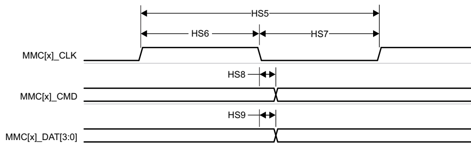
图 7-41. MMC1 - High Speed - Transmit Mode
